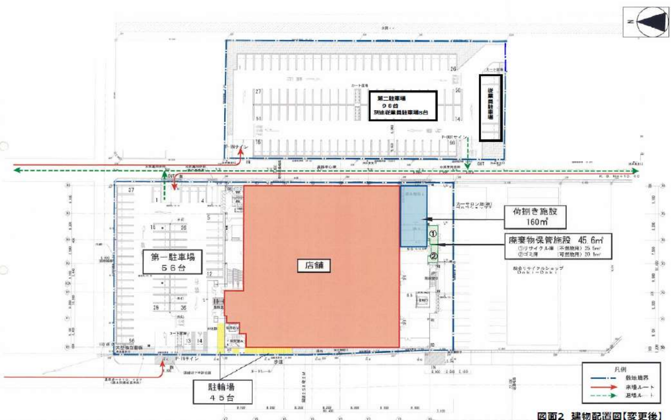
図面2 建物配置図【変更後】
