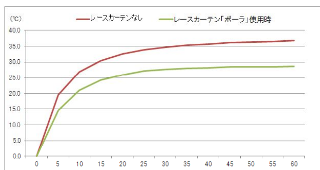
左:レースカーテン「ポーラ」製品使用イメージ 右:赤外ランプ 60°C法による室温上昇推移グラフ
