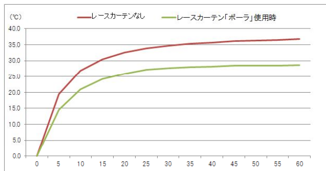
左:レースカーテン「ポーラ」製品使用イメージ 右:赤外線ランプ 60°C法による室温上昇推移グラフ
